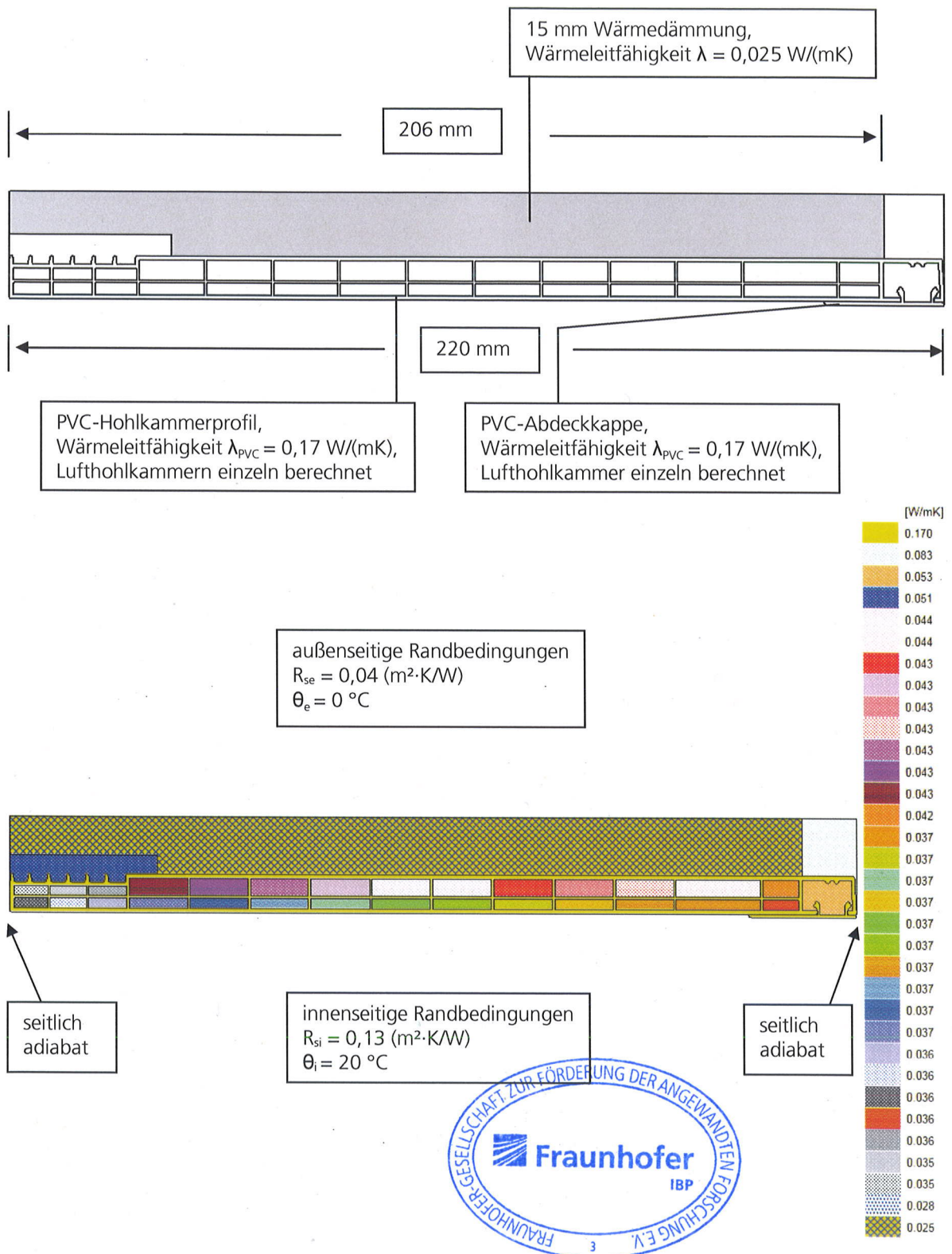
Bild 1: Oben: Berechnungsgeometrie auf Basis der Originalzeichnungsvorlage des Auftraggebers für das untersuchte Bauteil »Revileo® Rollkastendeckel mit Wärmedämmung 15 mm«. Unten: Berechnungsgeometrie mit Angabe der Wärmeleitfähigkeiten aller Materialien und Luftkammern sowie den klimatischen Randbedingungen für die thermische Simulation.
